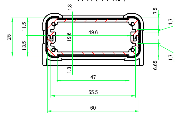
A-A (1:1.5)
